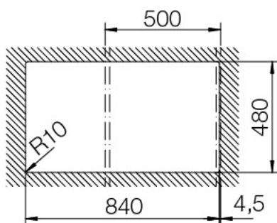
Maße für Einbau von oben
