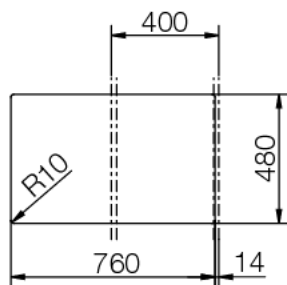
Maße für übergreifenden Einbau
